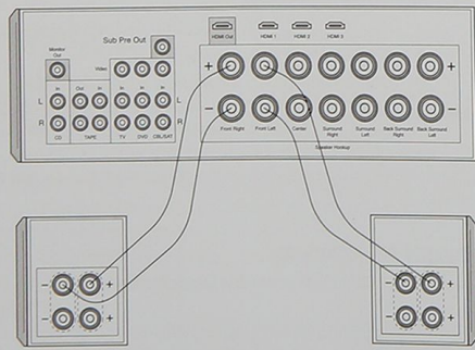
Figura 5 Conexiones estándar
