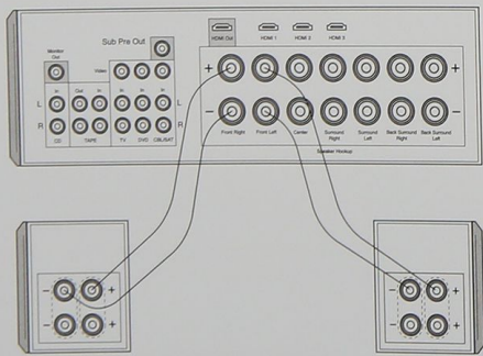
Figura 5 Conexões padrão
