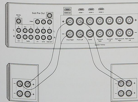
Abbildung 5 Standardanschlüsse
