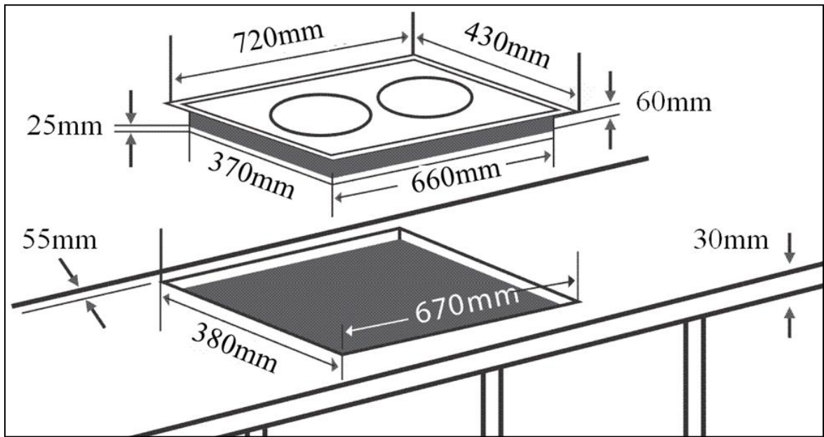
Kích thước khoét lỗ: EH-DIH220
