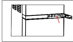
2. Kéo ống nhựa silicone ra.
