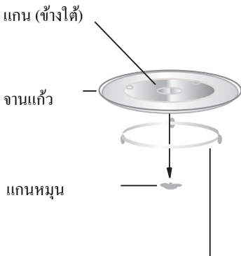
การประกอบจานหมุน
